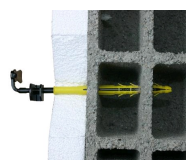
Arrêt de volet ISO - vue en coupe
