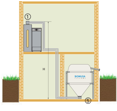
SYSTÈME D'ALIMENTATION POUR SILO ARTISANAL AVEC UNITÉ DE COMMUTATION SUR COLLECTEURS D'ASPIRATIONS
