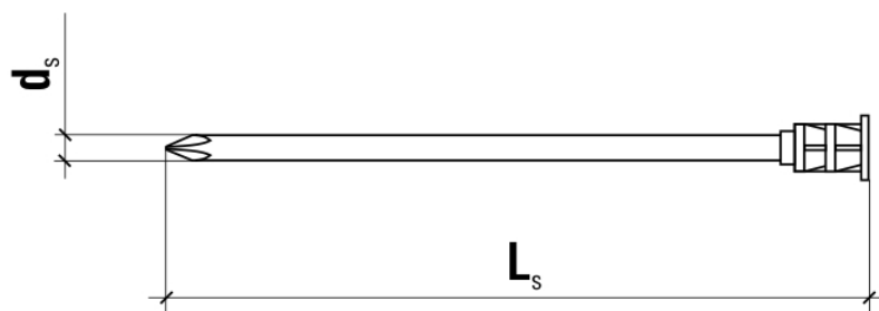
Clou spécial d'expansion TMX-4,4
