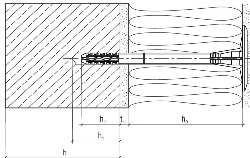
montage de surface
