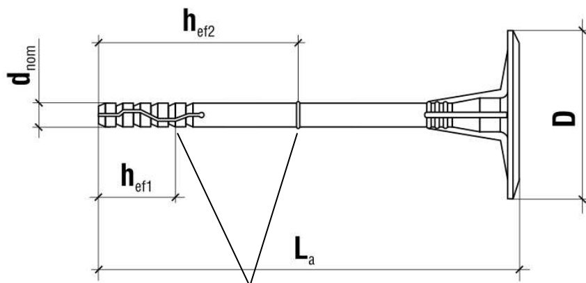
Marquage de la profondeur d'ancrage
