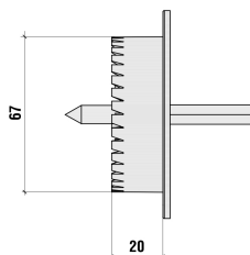
Fraise du plastique WK-FT pour le montage profond
