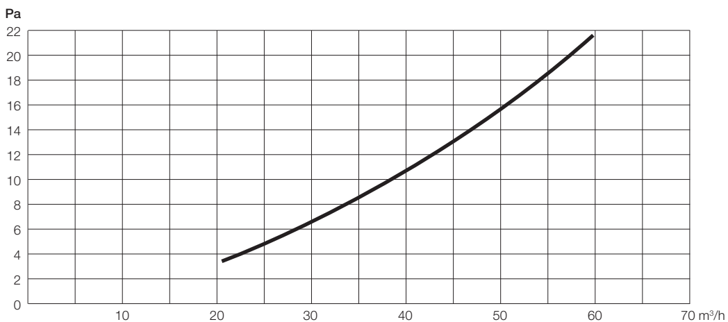
Perte de charge de la grille ronde design Zehnder Venezia DN125, blanc
