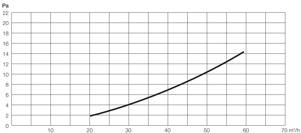
Perte de charge de la grille ronde design Zehnder Torino DN125, inox
